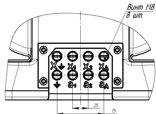
Рисунок А.2 Клемник для трансформаторов ЗНОЛ-35 III (остальное см. рисунок А.1, крышка условно не показана)
