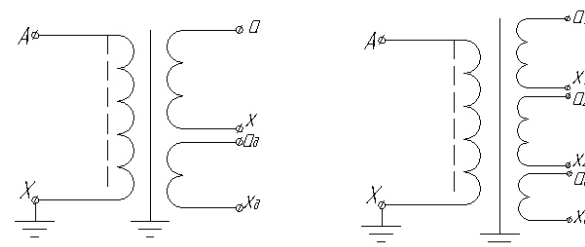
Рисунок А.3 Принципиальная электрическая схема трансформатора ЗНОЛ-35(27) III
